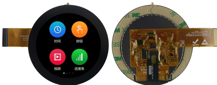
图 1-1 2.1 寸电容触摸参考图
